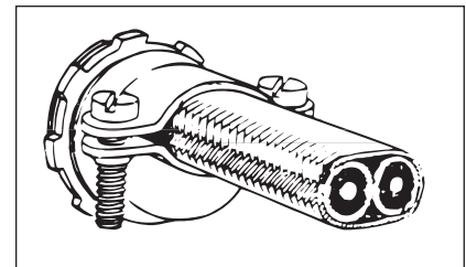
Installation type (câble sous gaine non métallique)
