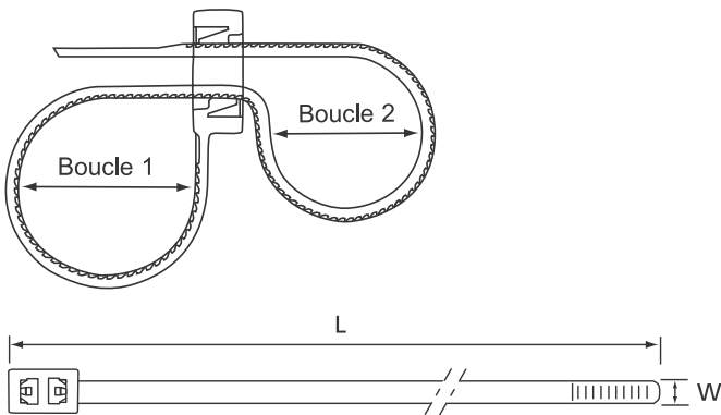
L'attache à boucle double Ty-Fast md permet de réunir en parallèle deux faisceaux de câbles avec une seule attache pour câbles. Disponible en 3 longueurs différentes.
